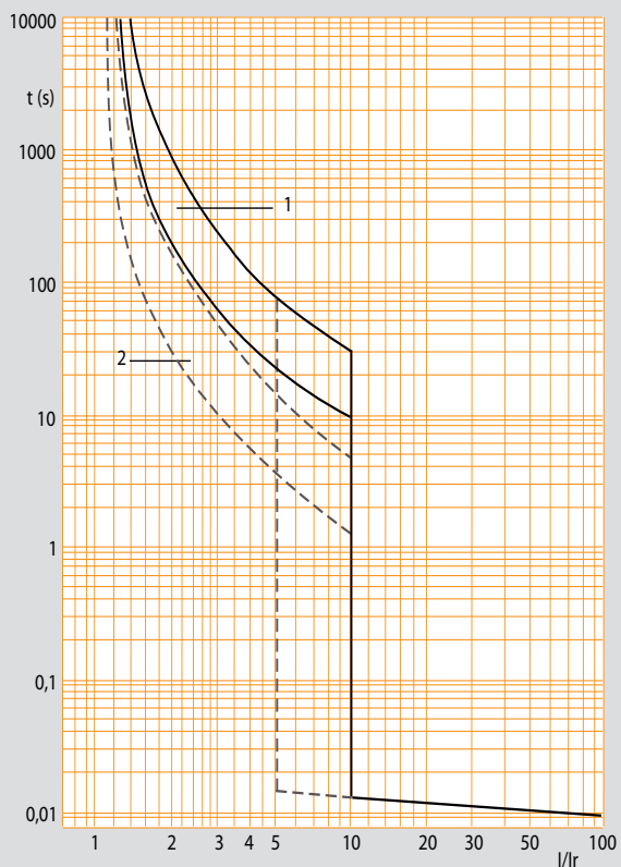
TIEMPO-CORRIENTE
